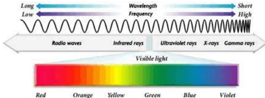
Espectro electromagnético
